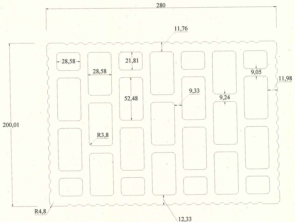
Σχήμα 1. Γεωμετρία οπτόπλινθου
